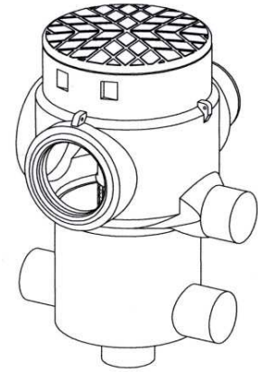
Anlieferzustand: Maxi Plus vormontiert
